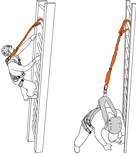
K.2 - Sırttan Kullanım A Ankraj Noktası (Şekil- 3.2) Use of Dorsal A Attachment Point (Figure-3.2)
