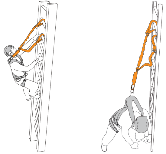
H.2 - Sırttan Kullanım A Ankraj Noktası (Şekil - 1.2) Use of Dorsal A Attachment Point (Figure -1.2)
