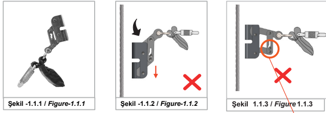
Şekil -1.1.2 / Figure-1.1.2 - Şekil -1.1.3 / Figure-1.1.3. (TR) SRG-1 A üzerindeki pin, ters çevildiğinde aşağı düşmekte ve SRG-1 A'nın halata ters takılmasını engellemektedir. (EN) When the user tries to put the SRG-1 A Energy Absorber Rope Grabe upside down, the pin on the SRG-1 A is dropping down and avoiding it to be put on the line. Figure-1.1.3
