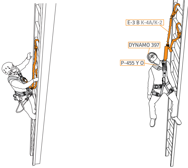
LANYARDIN GÖĞÜSTEN A ANKRAJ NOKTASINA BAĞLANARAK KULLANIMI
