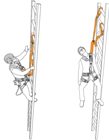
J.1 - Göğüsten Kullanım A Ankraj Noktası (Şekil - 3.1) Use of Sternal A Attachment Point (Figure -3.1)
