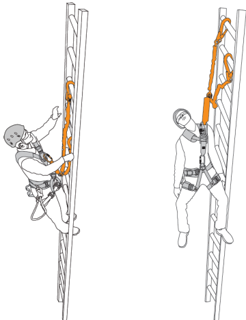
I.1 - Göğüsten Kullanım A Ankraj Noktası (Şekil-2.1) Use of Sternal A Attachment Point (Figure-2.1)
