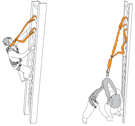
I.2 - Sırttan Kullanım A Ankraj Noktası (Şekil-2.2) Use of Dorsal A Attachment Point (Figure-2.2)
