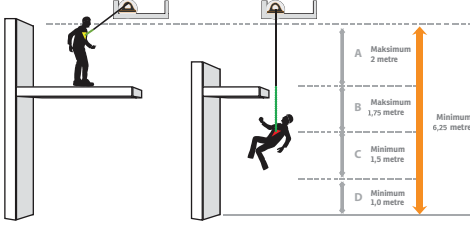
(TR) Güvenli Açık Düşüş Mesafesi = A+B+C+D (EN) Fall Clearance = A+B+C+D
