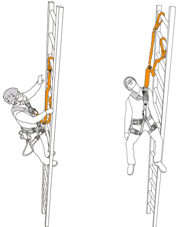
H.1 - Göğüsten Kullanım A Ankraj Noktası (Şekil- 1.1) Use of Sternal A Attachment Point (Figure-1.1)
